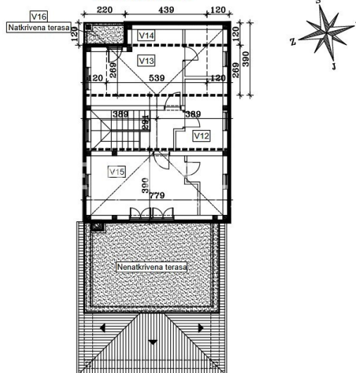
TLOCRT KATA
